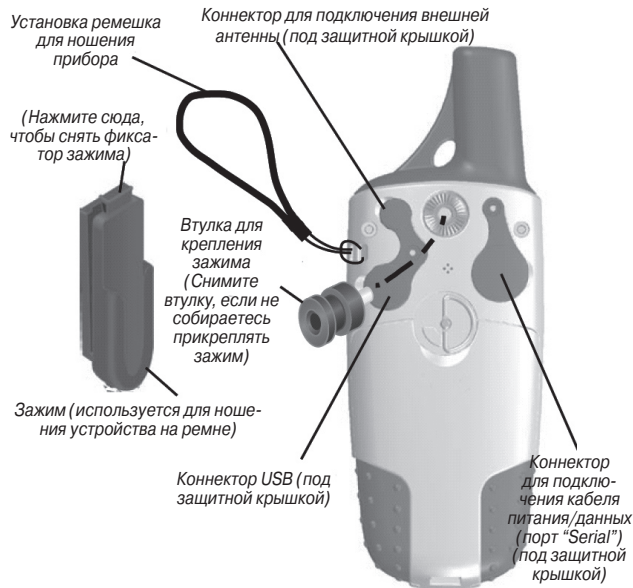
Вид сзади прибора GPSPар 60
